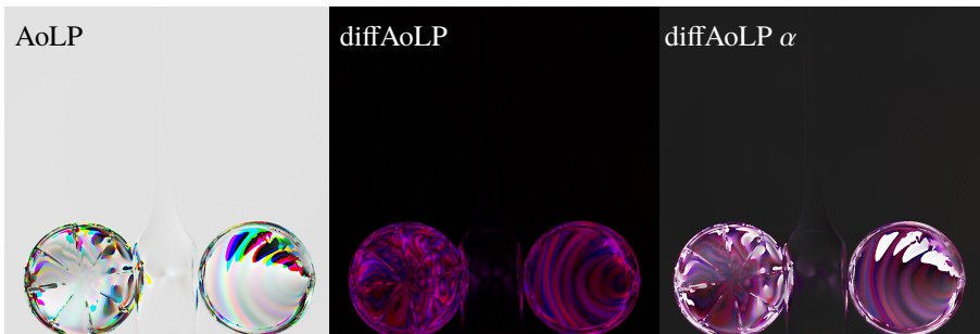
ours
